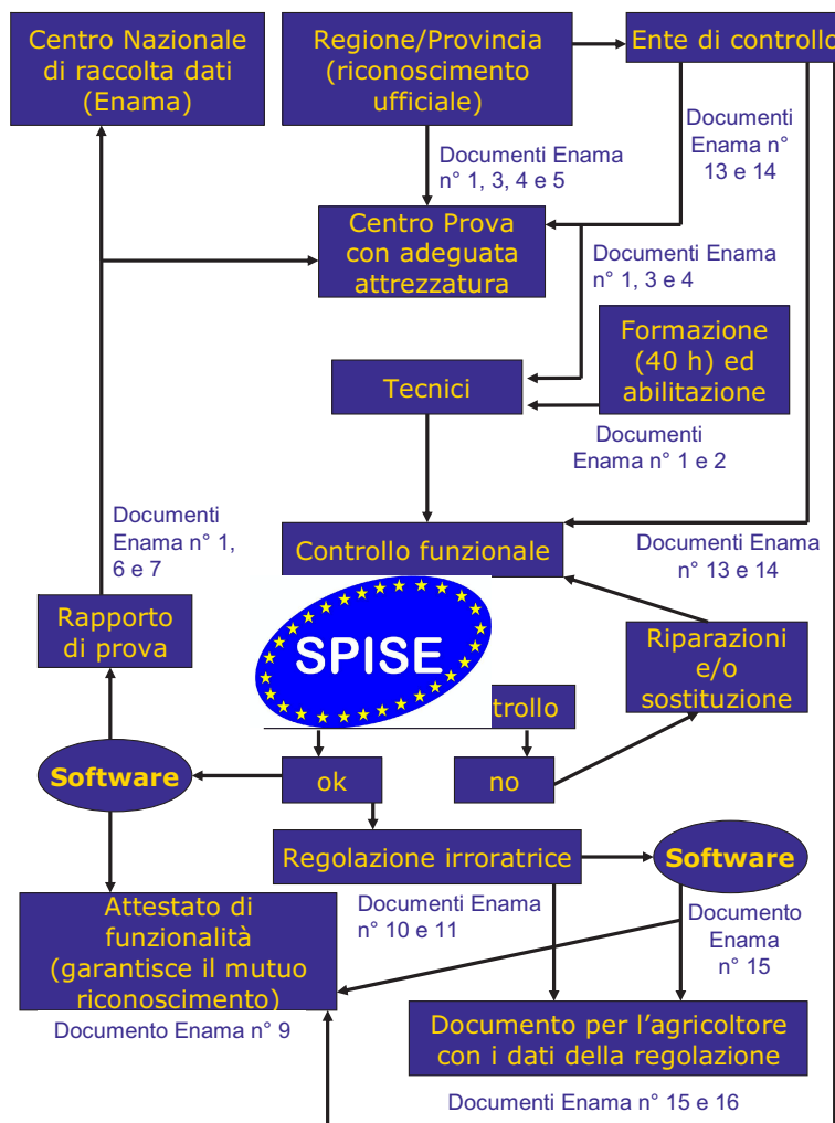
Fig. 2 – Schema dell’organizzazione del servizio di controllo funzionale e regolazione delle macchine irroratrici secondo quanto previsto dal Gruppo di Lavoro ENAMA.
