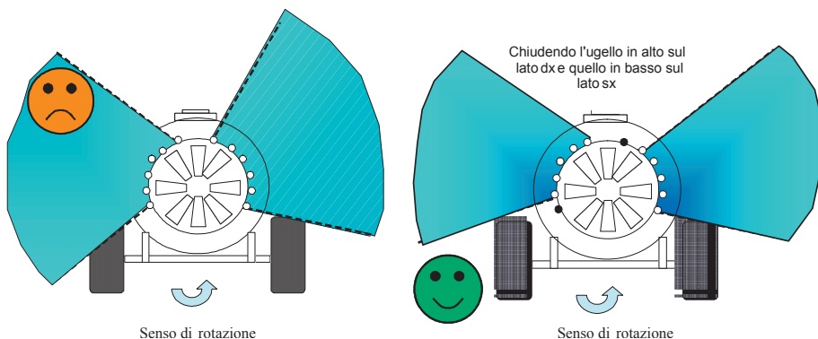
Figura 5 - Nelle irroratrici con ventilatore assiale chiudendo l'ugello in alto sul lato sinistro e quello in basso sul lato destro è spesso possibile uniformare il profilo dello spray sui due lati della macchina.
