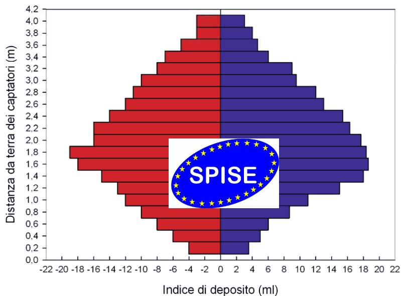
Figura 17 – Esempio di diagramma di distribuzione misurato su entrambi i lati della macchina irroratrice.
