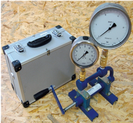
Fig. 3 - Esempio di banco prova per la valutazione della funzionalità del manometro (foto - DEIAFA).
