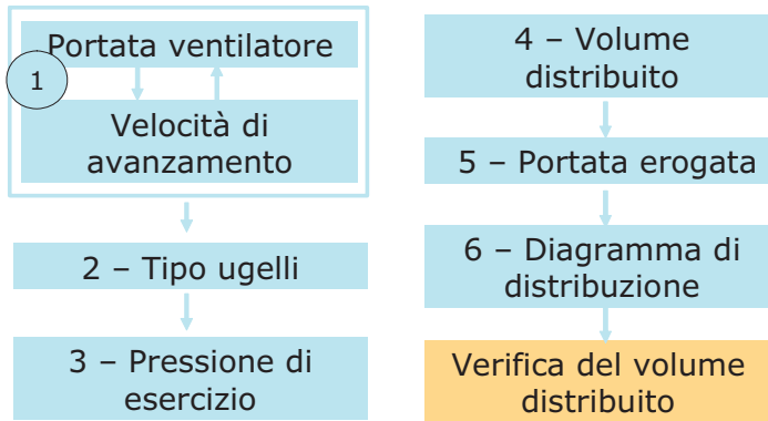
Figura 2 - Ordine di esecuzione delle regolazioni della macchina irroratrice.
