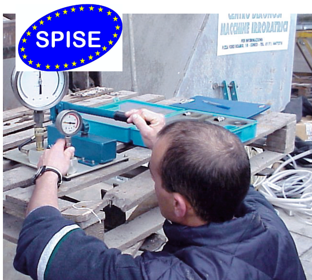
Fig. 12 – Verifica funzionalità del manometro (foto G. Oggero – DEIAFA)
