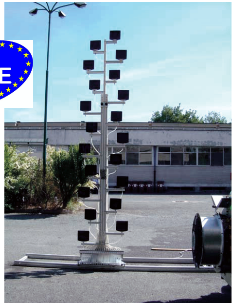
Fig. 6 - Esempio di banco verticale a vassoi rettangolari per la determinazione del diagramma di distribuzione di una irroratrice per colture arboree (foto G. Oggero - DEIAFA).
