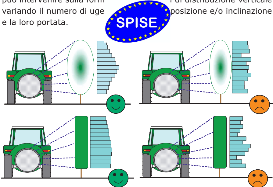
Figura 4 - Adeguamento del diagramma di distribuzione alla forma di allevamento e allo spessore della vegetazione.
